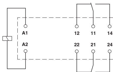
Электрическая схема
