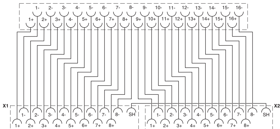
Электрическая схема
