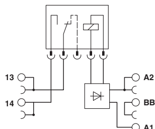
Электрическая схема
